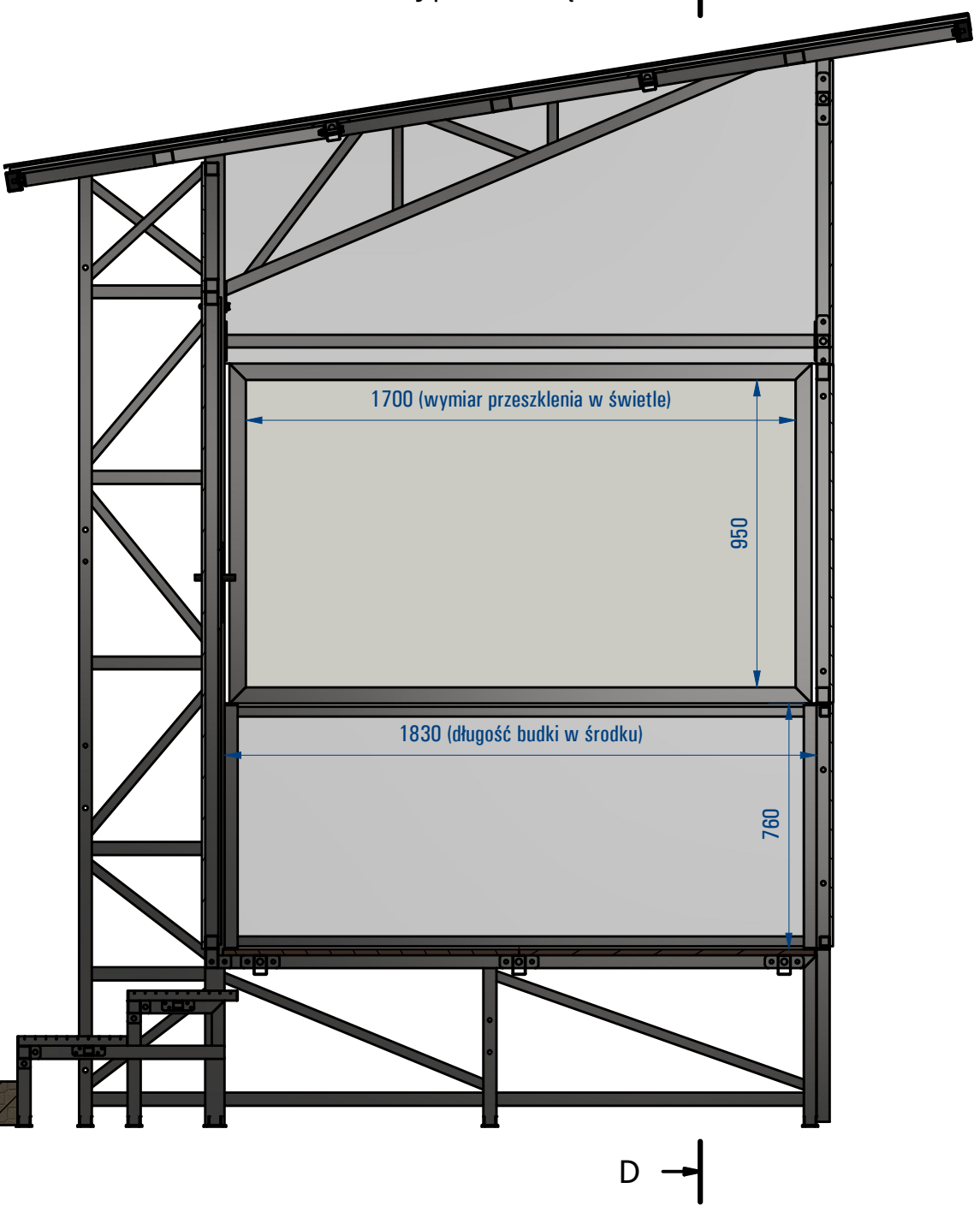
C-C ( 1 : 20 ) Przekrój przez budkę D →
